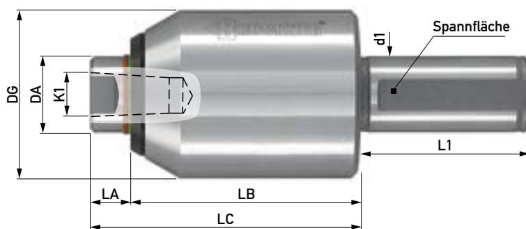
Zentriereinsätze für Typ TRE Seite 35
