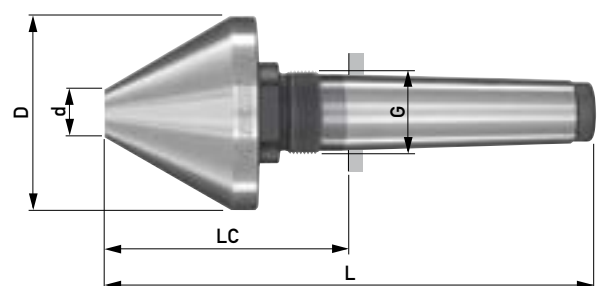
Form 258 Zentrierkegel 60°
