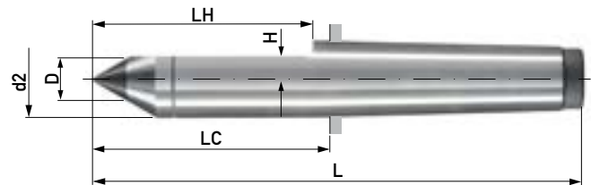
Form HL größerer Hartmetall-Ø DIN-Länge und verlängert
