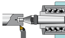
Form 257 zum Gewindedrehen und für tieferliegende Zentren
