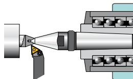
Form 256 bei beengtem Arbeitsraum
